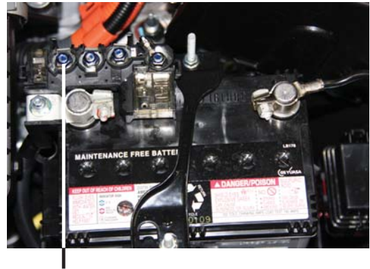
Connexion du câble du convertisseur c.c. à c.c.
